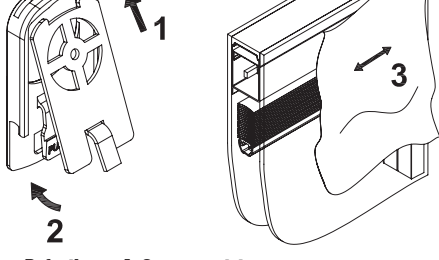
Befestigung Außenmagnetsteuerung
